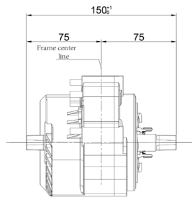
Mid-aandrijf motor
